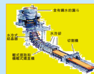
典型的連續澆鑄示意圖
