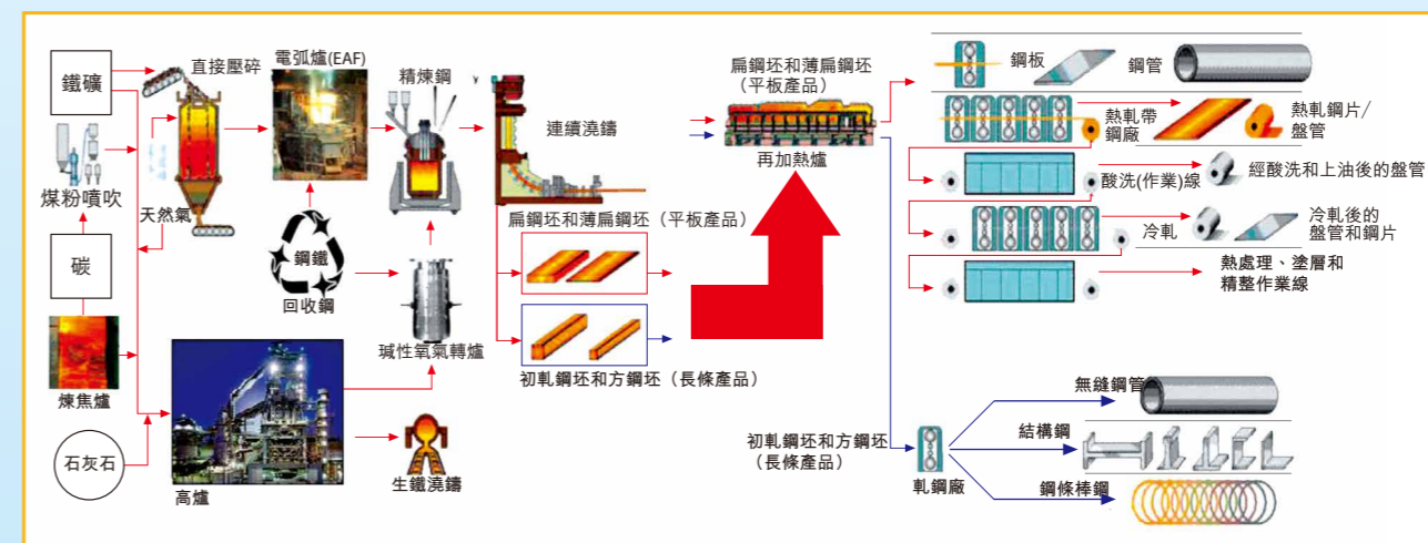
一家綜合煉鋼廠的生產過程（從熔區到軋鋼廠）
